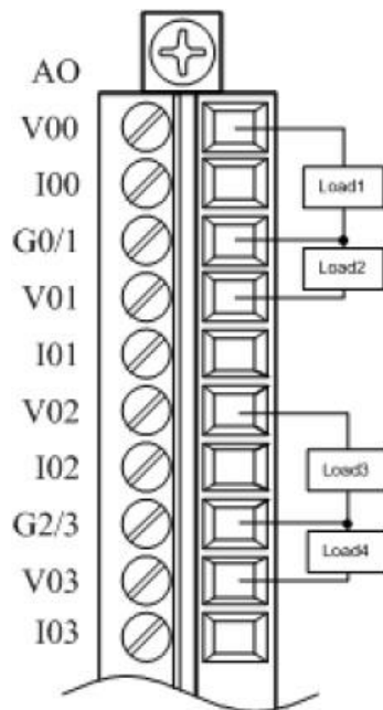
전압 신호
